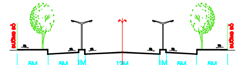
MẶT CÁT 1-1 (ĐƯỜNG LỀ VÂN TÂM (ĐƯỜNG QUỐC LỘ 54))
