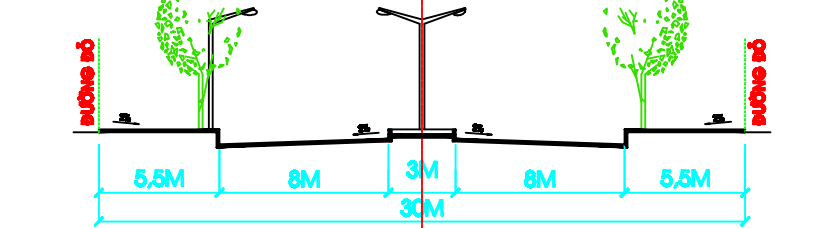
MẶT CÁT 2-2
