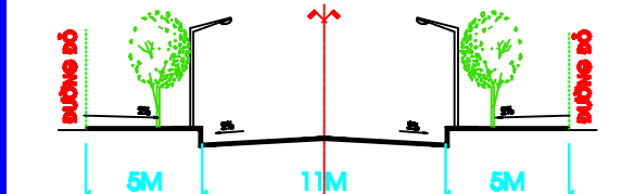
MẶT CÁT 5-5
