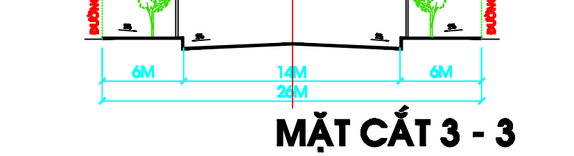
MẶT CÁT 3-3
