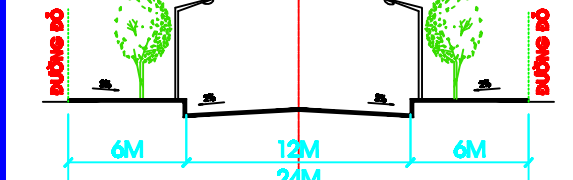
MẶT CÁT 4-4 (ĐƯỜNG ĐỒNG KHỚP NỐI DÀ)
