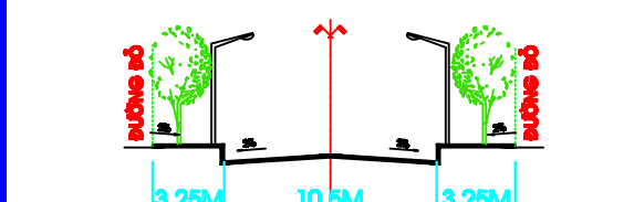
MẶT CÁT 6-6
